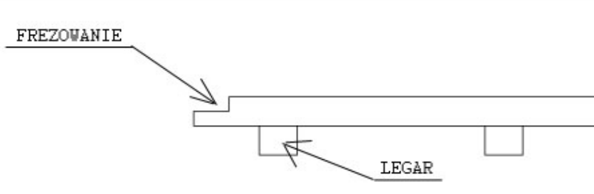
Rys.3 Przekrój podłużny blatu podłogowego
