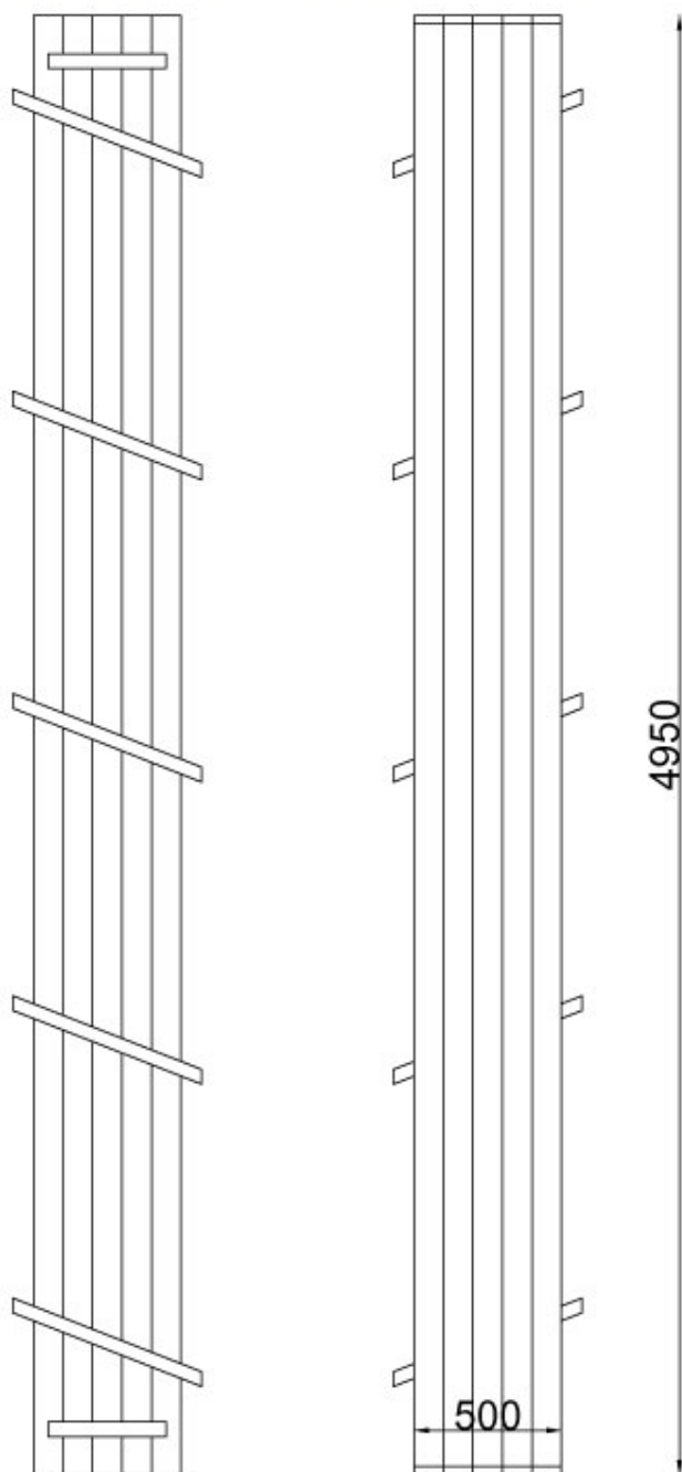
Rys.4 Widok z dołu i widok z góry blatu podłogowego
